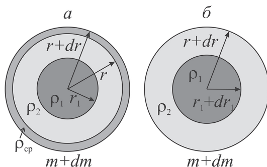
Рис. 2. Дифференциация в процессе роста шара: а – увеличение текущей массы шара m на dm , б – конфигурация шара массы m = dm после дифференциации
